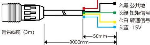
插口管脚分配
